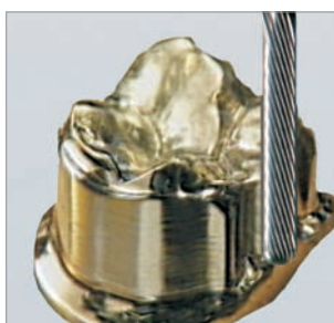
Fresaggio parallelo di una corona di metallo. Fresado paralelo de una corona metálica. Fresagem paralela de coroa metálica.
